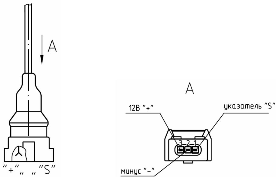
Рисунок 7.14.1– Схема подключения ДОТ.4 к трехконтактной колодке жгута
