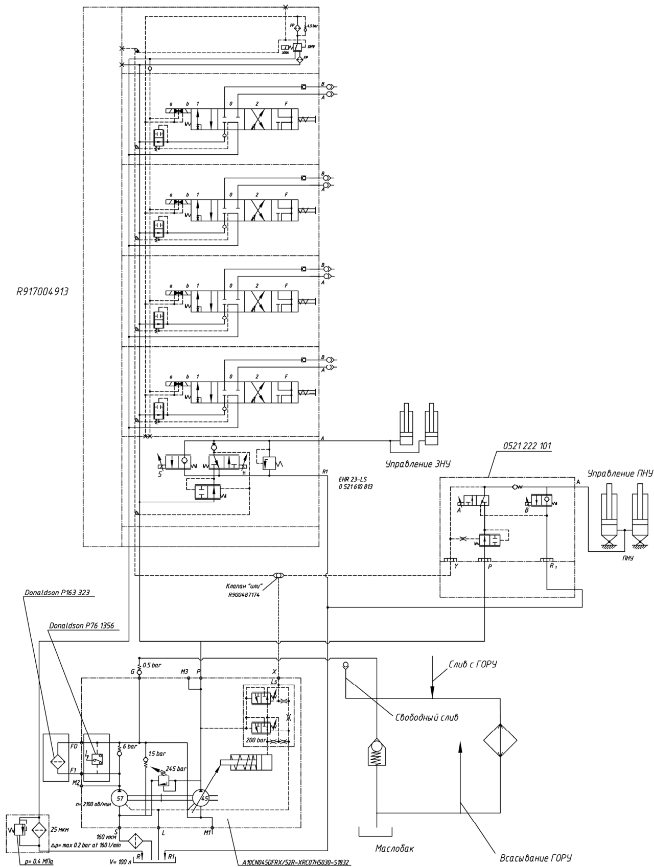
Рисунок 3.16.4 – Принципиальная гидравлическая схема ГНС
