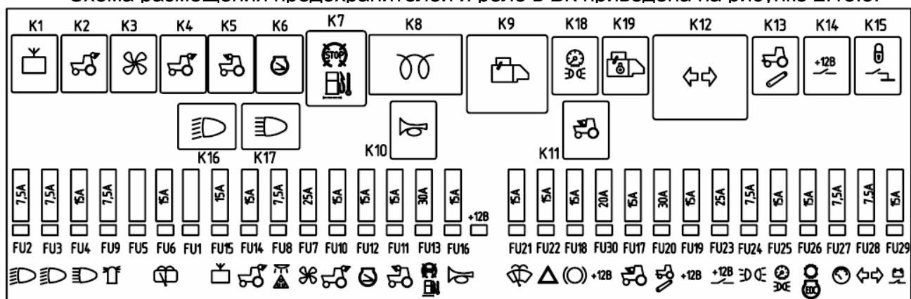
Рисунок 2.18.3 – Схема размещения предохранителей и реле в БК
