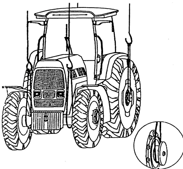
Рисунок 9.1.1 – Схема строповки трактора
